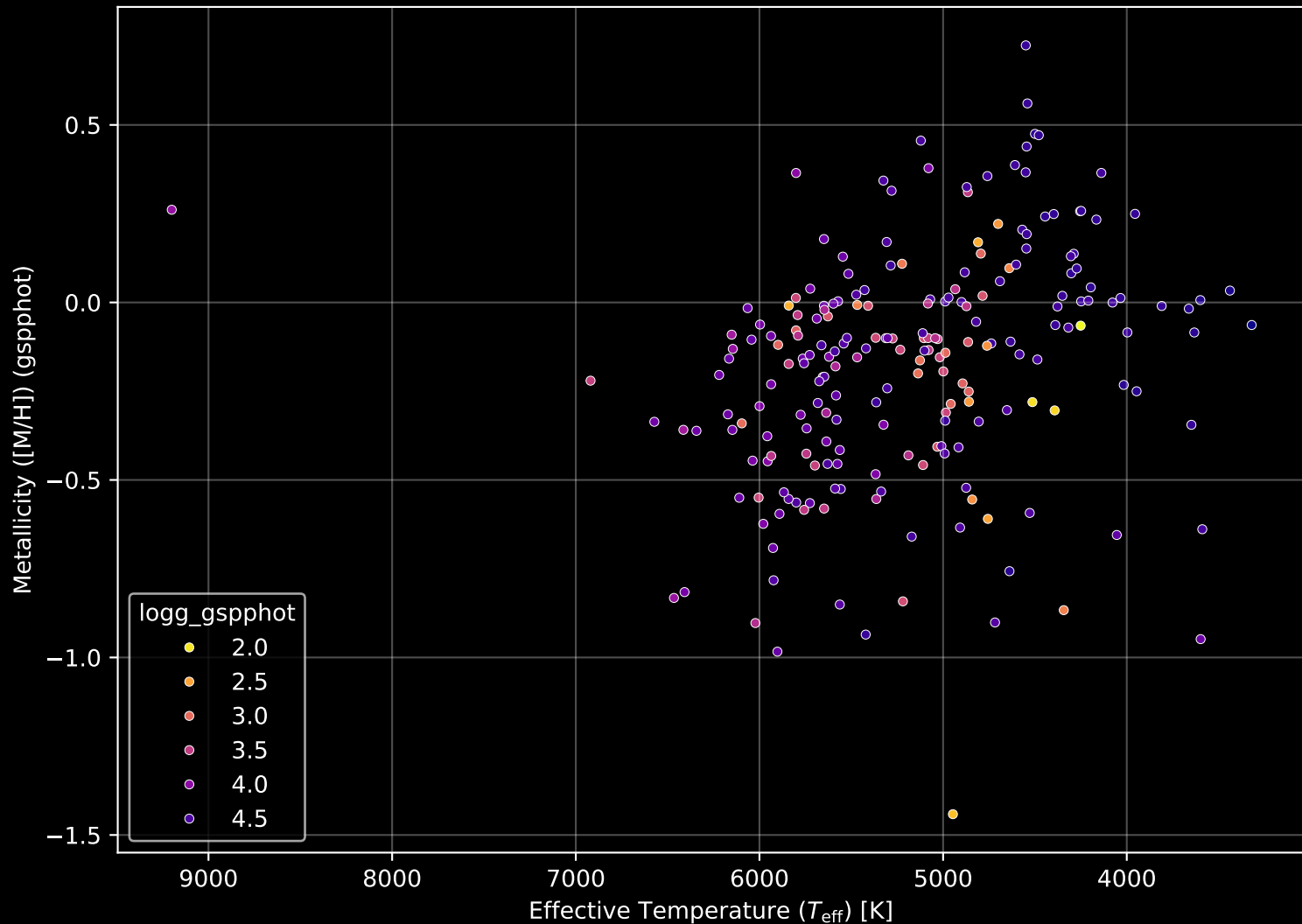
APOGEE DR17 Field: [209+73_btx] Stellar Population Parameters (n= 216)
